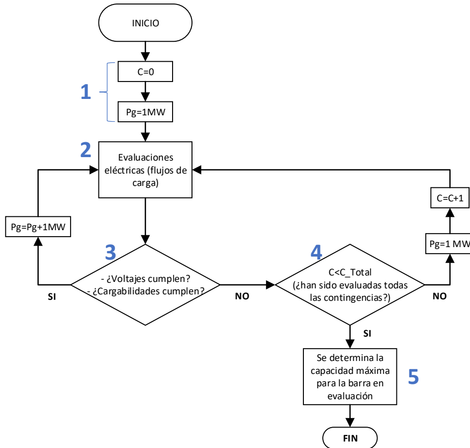
Figura 5-1 Diagrama de flujo del cálculo de la capacidad por nodo
