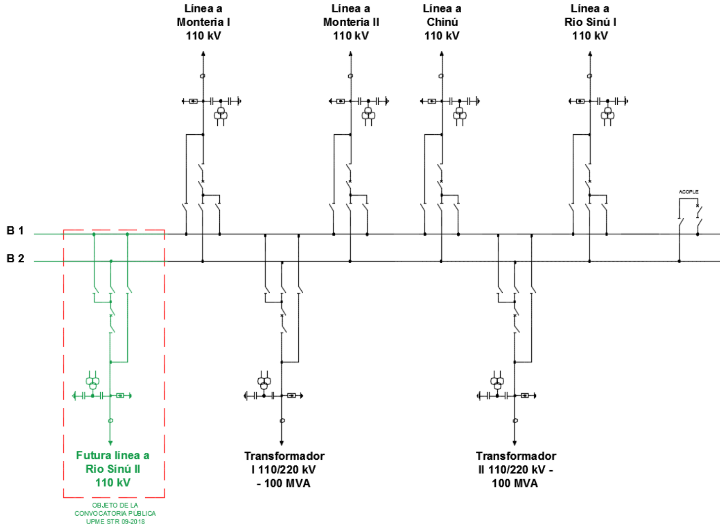
Figura 3 – SE Nueva Montería 110 kV (PREPUBLICACIÓN)
