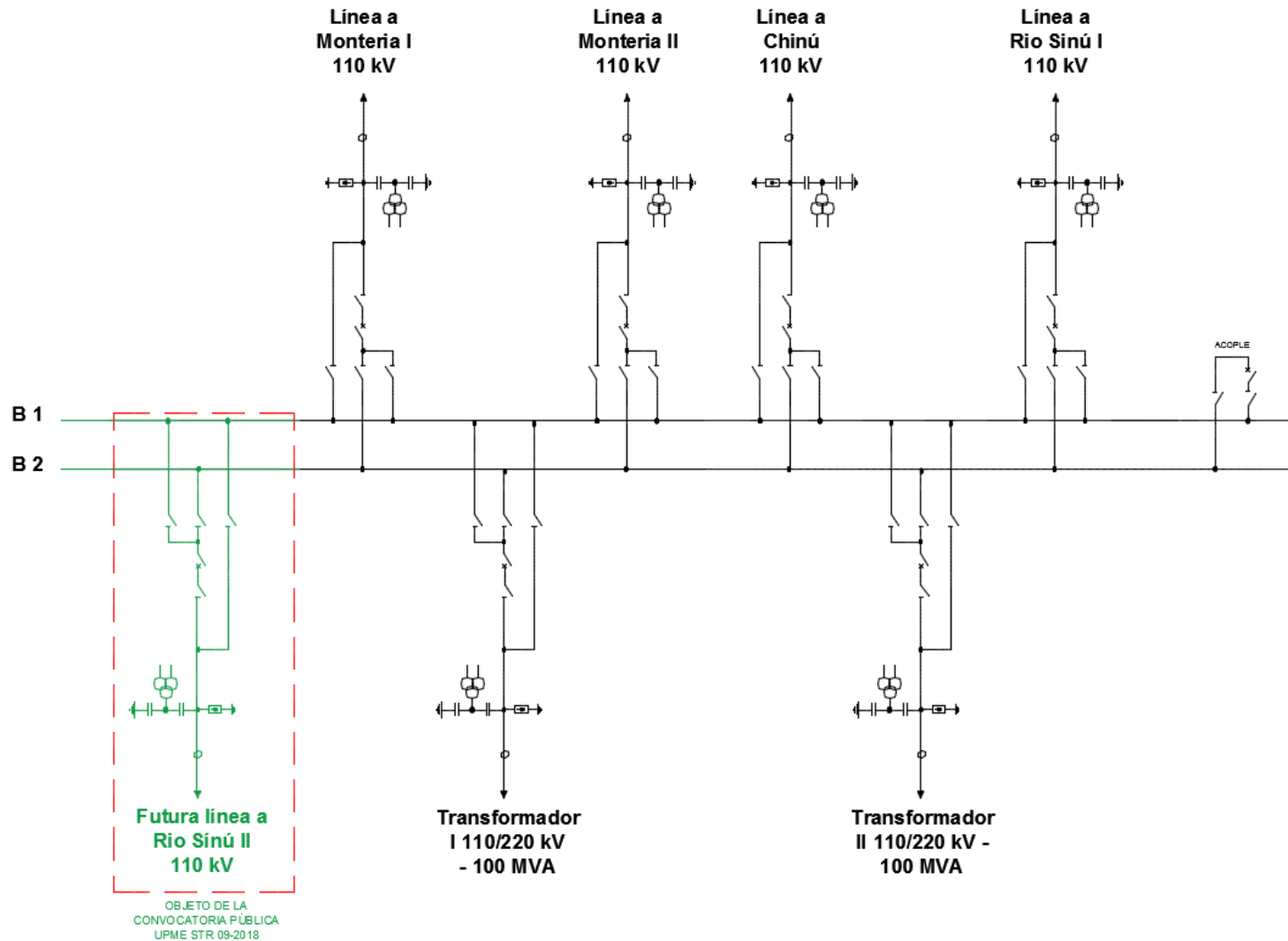
Figura 3 – SE Nueva Montería 110 kV
