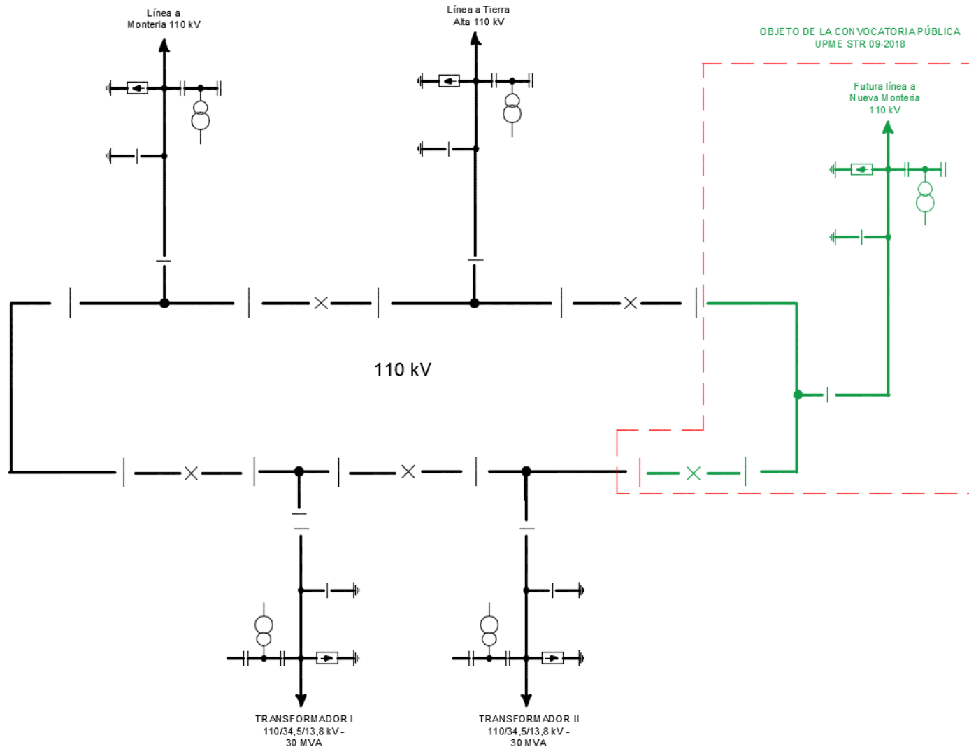
Figura 2 – SE Rio Sinú 110 kV
