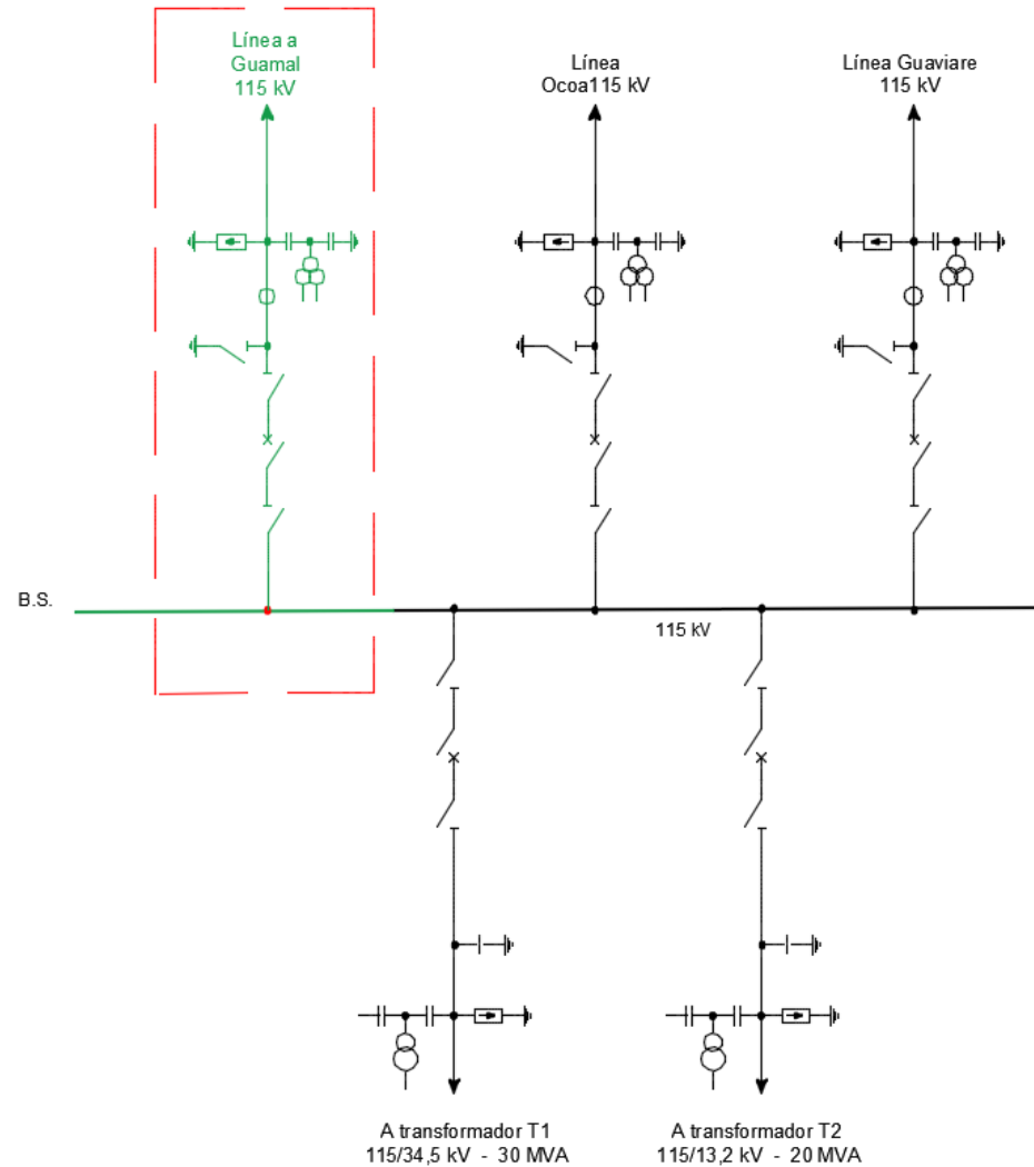
Figura 2 – SE Granada 115 kV (PREPUBLICACIÓN)
