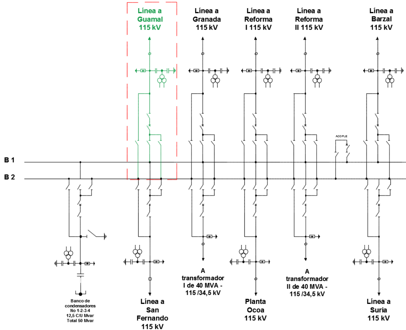
Figura 3 – SE Ocoa 115 kV (PREPUBLICACIÓN)
