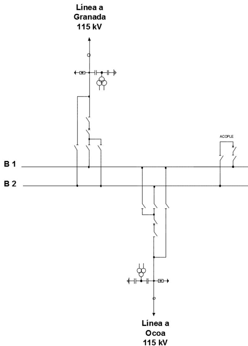
Figura 2 – SE Guamal 115 kV (PREPUBLICACIÓN)
