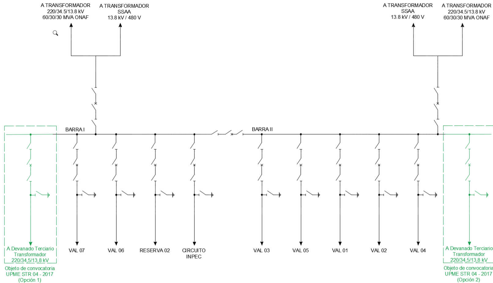
FIGURA 2. SUBESTACIÓN VALLEDUPAR 13.8 kV
