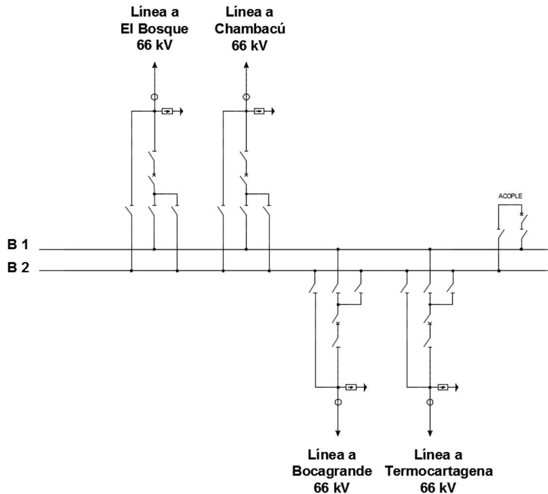
FIGURA 2 - SUBESTACIÓN LA MARINA 66 kV
