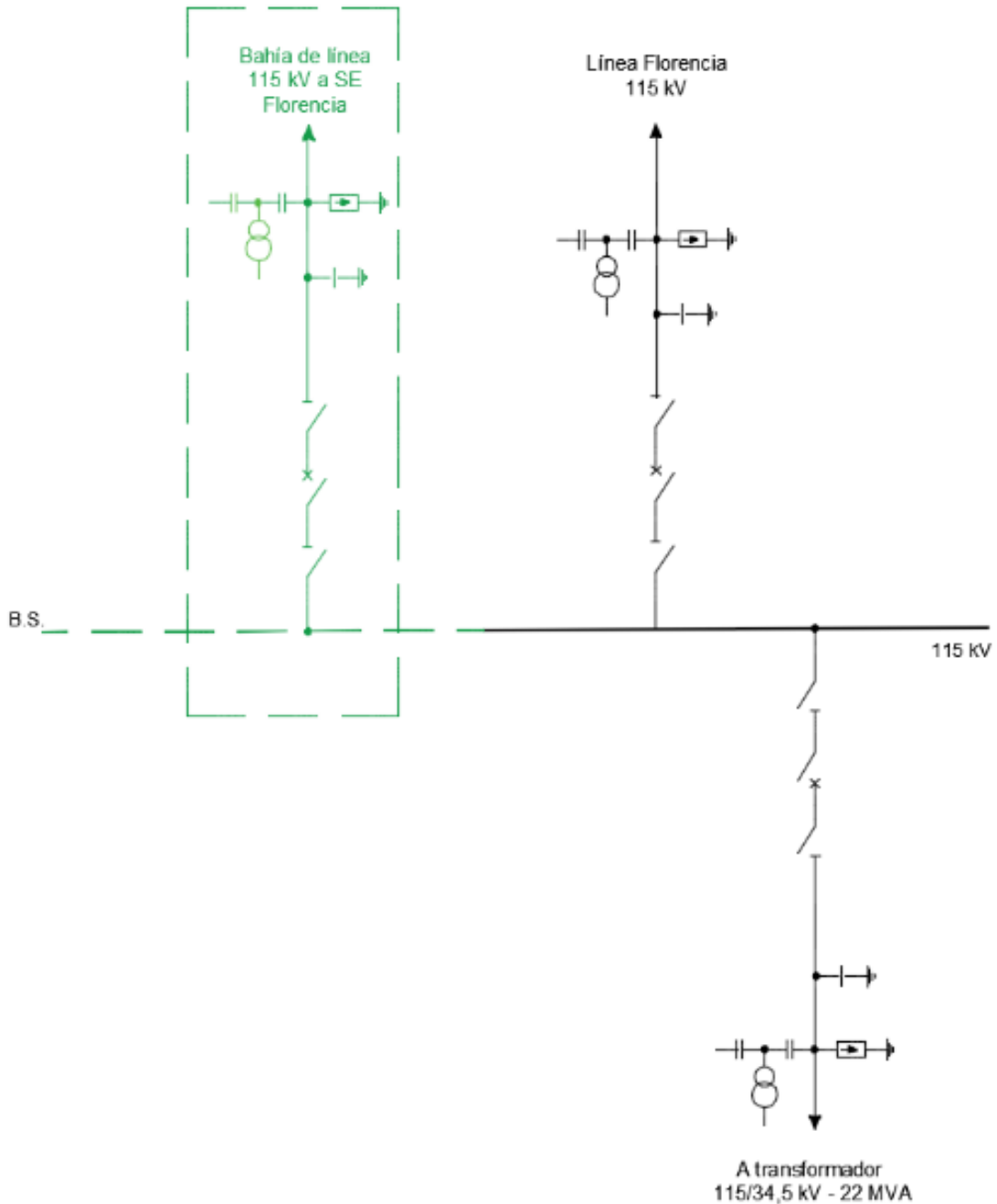
FIGURA 4. ESQUEMA UNIFILAR SUBESTACIÓN DONCELLO 115 kV
