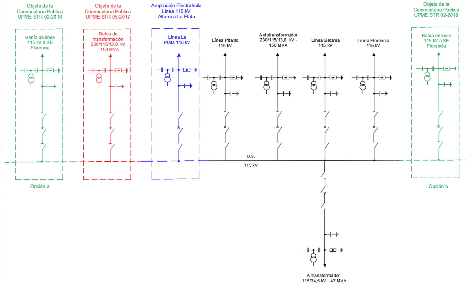
Diagrama Unifilar SE Altamira 115 kV
