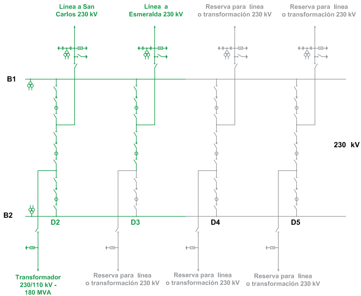
Figura 2. Diagrama Unifilar San Lorenzo 230 kV (Prepublicación)
