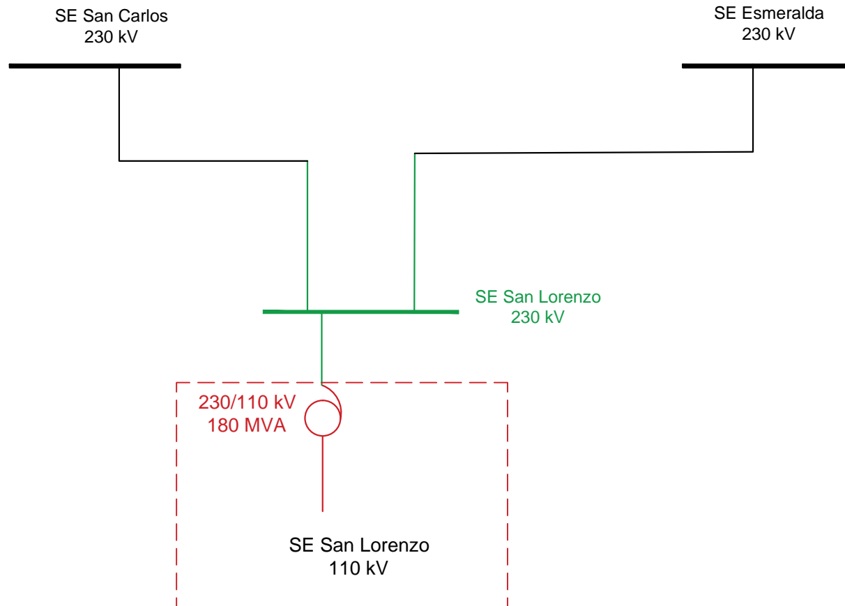
Figura 1. Diagrama esquemático San Lorenzo 230 kV (Prepublicación)
