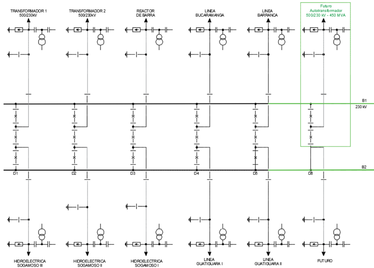
Figura 2 - Diagrama Unifilar Subestación Sogamoso 230 kV (PREPUBLICACIÓN)
