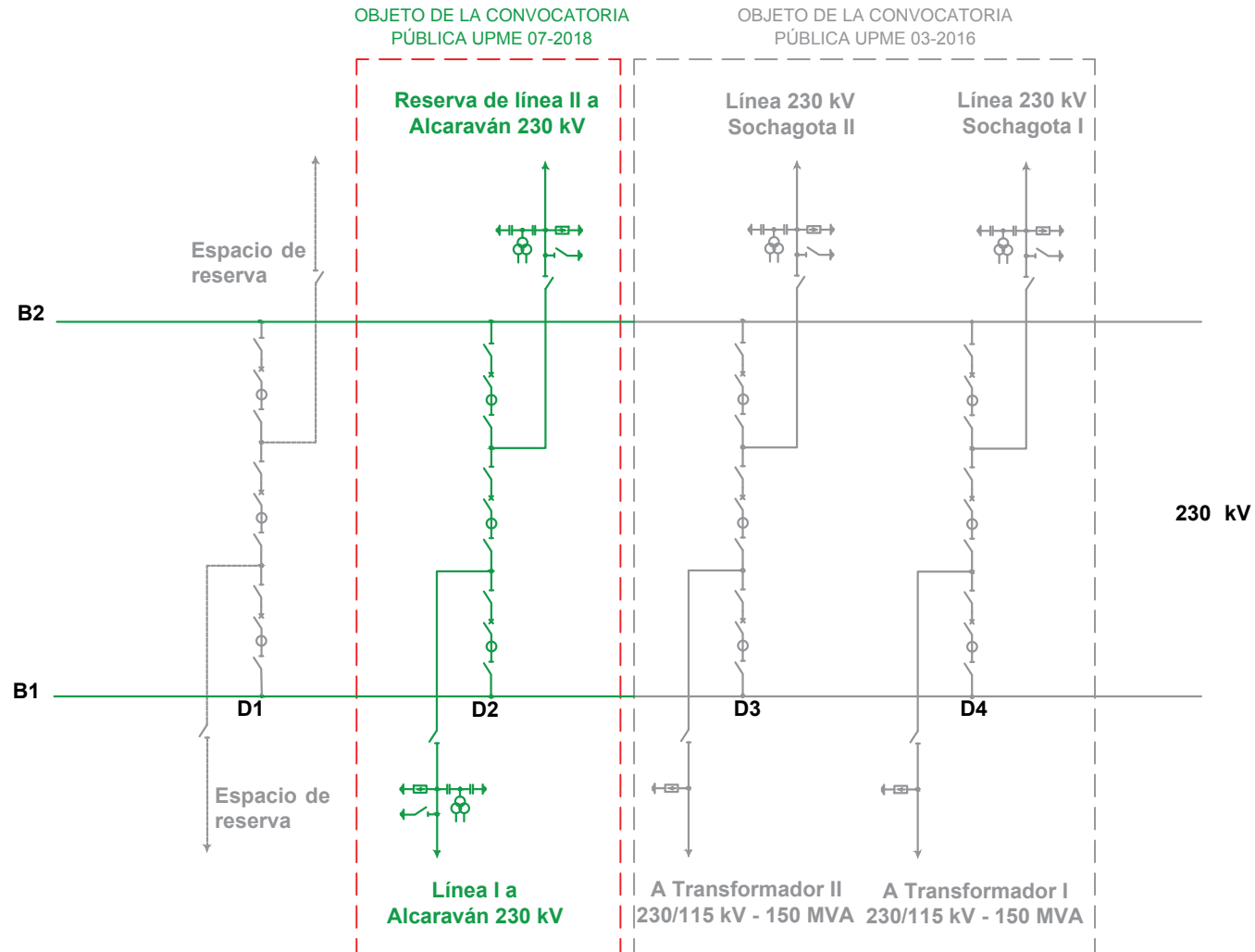
Figura 3. Diagrama Unifilar Subestación San Antonio 230 kV (Prepublicación)
