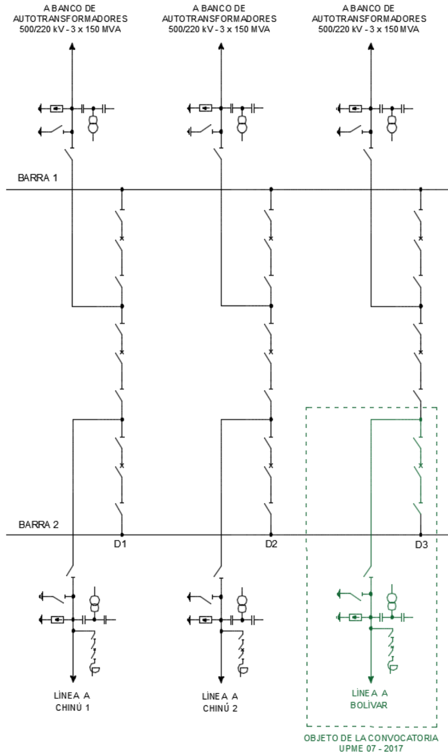
FIGURA 2. SUBESTACIÓN SABANALARGA 500 kV (PREPUBLICACIÓN)
