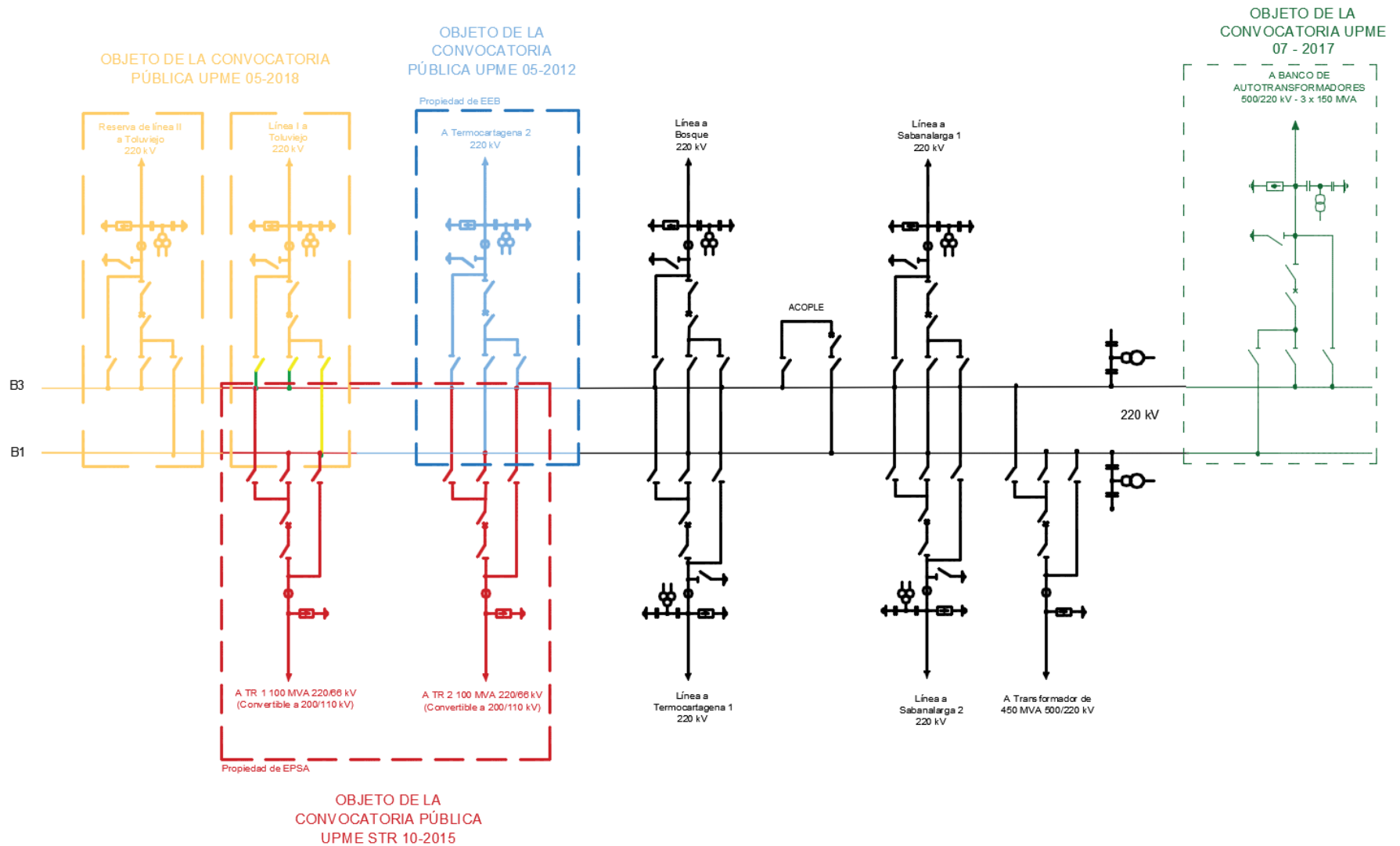
FIGURA 4. SUBESTACIÓN BOLÍVAR 220 kV
