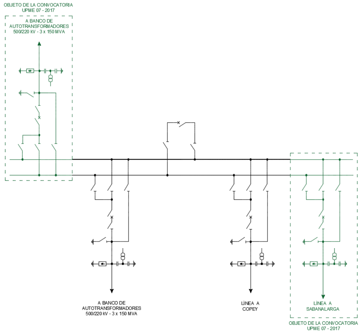
FIGURA 3. SUBESTACIÓN BOLÍVAR 500 kV
