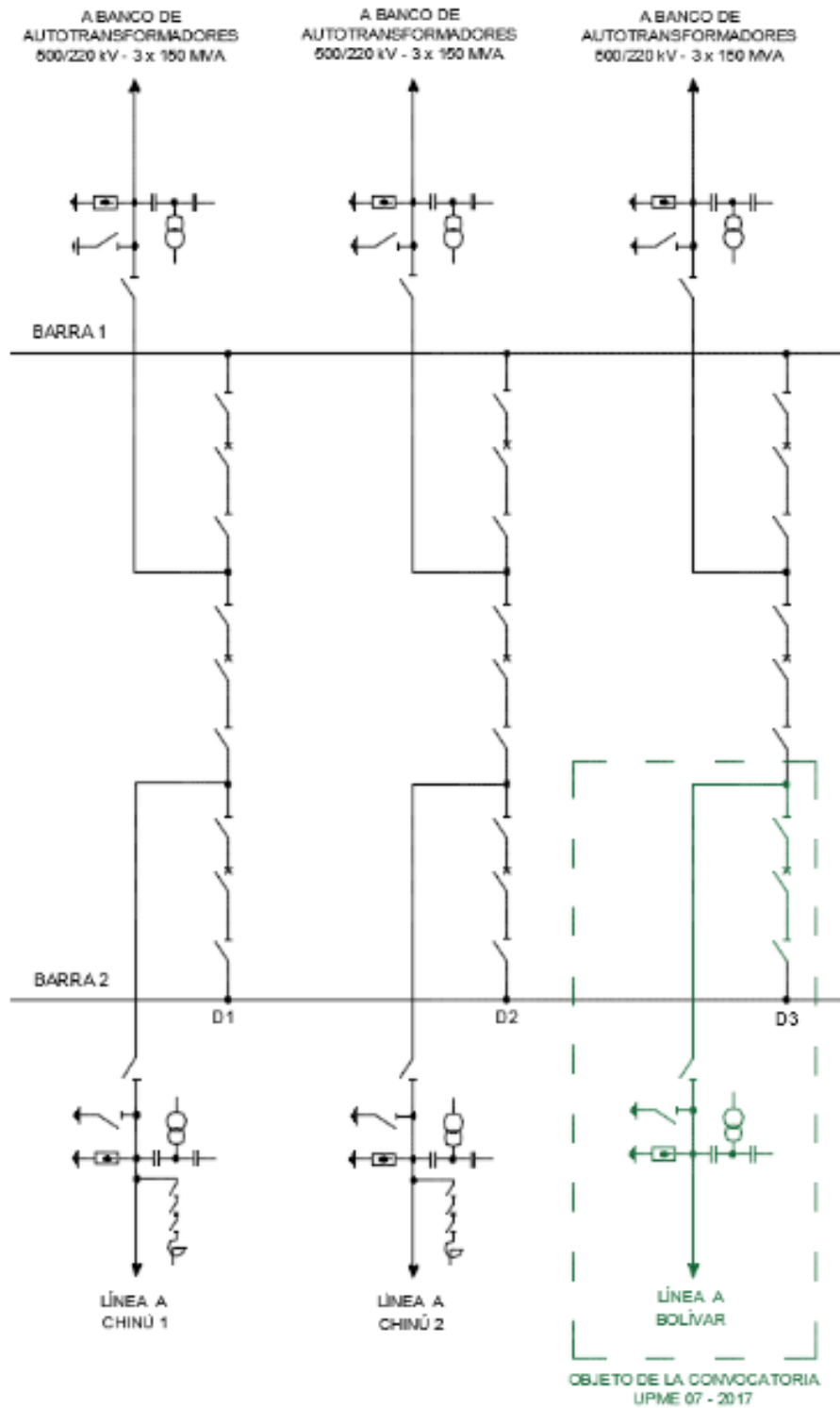
FIGURA 2. SUBESTACIÓN SABANALARGA 500 kV
