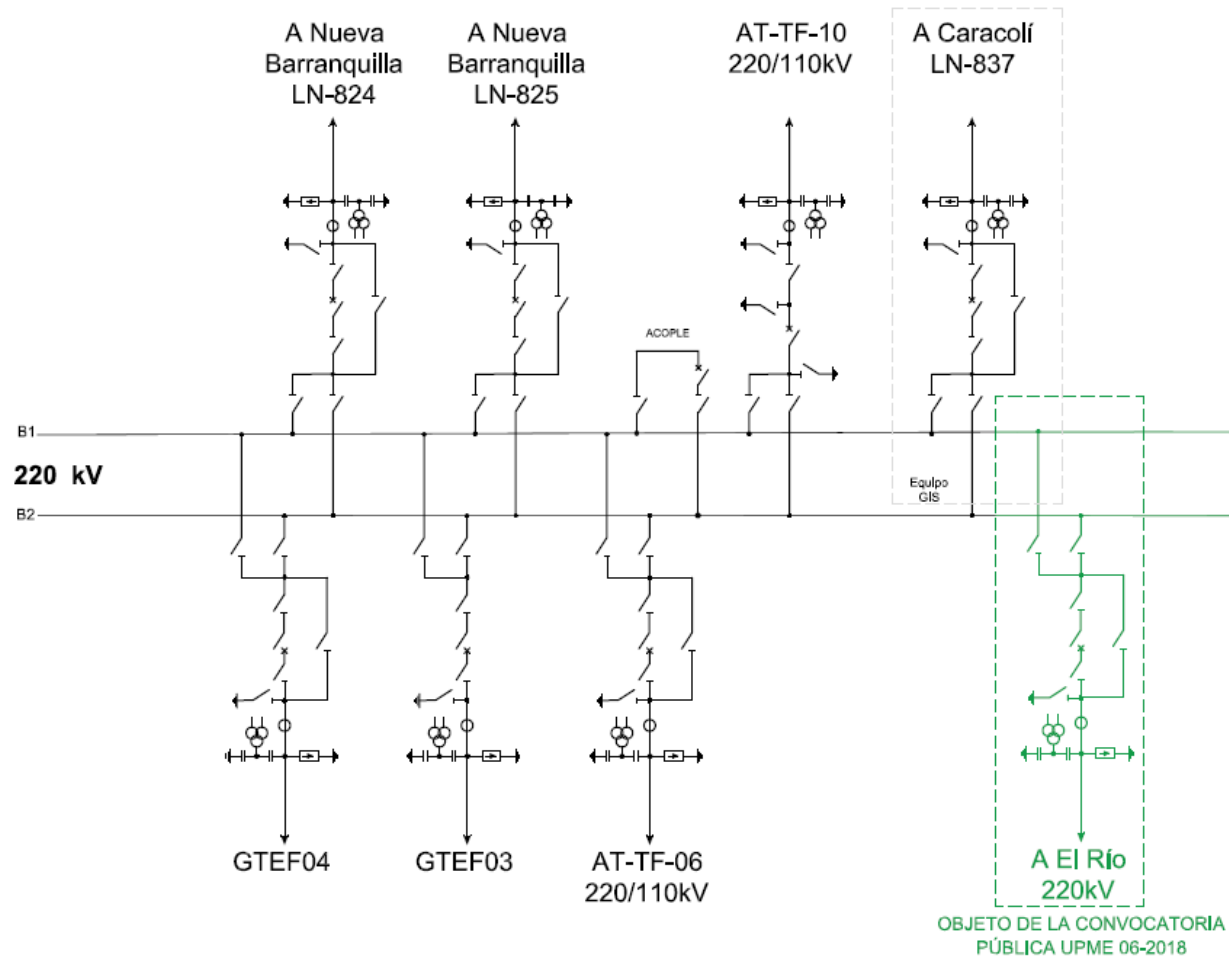
FIGURA 3 - ESQUEMA UNIFILAR SUBESTACIÓN TERMOFLORES 220kV (PREPUBLICACIÓN)
