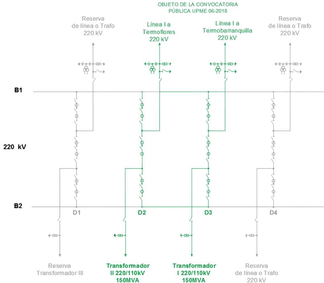
Figura 2 - Diagrama Unifilar Subestación El Rio 220 kV
