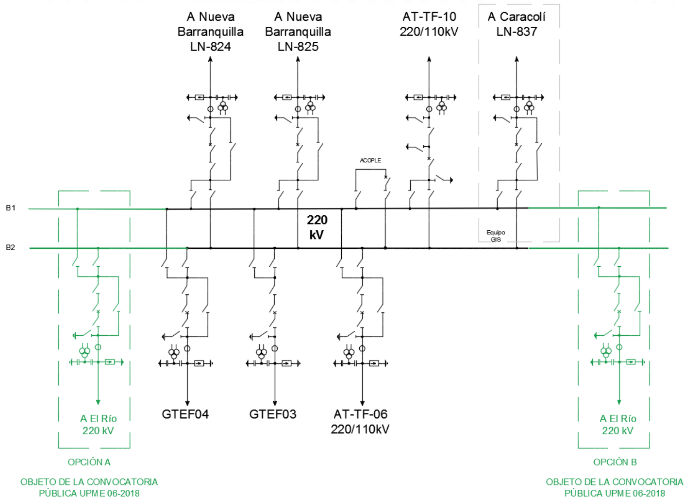
Figura 4 - Diagrama Unifilar Subestación Termoflores 220 kV
