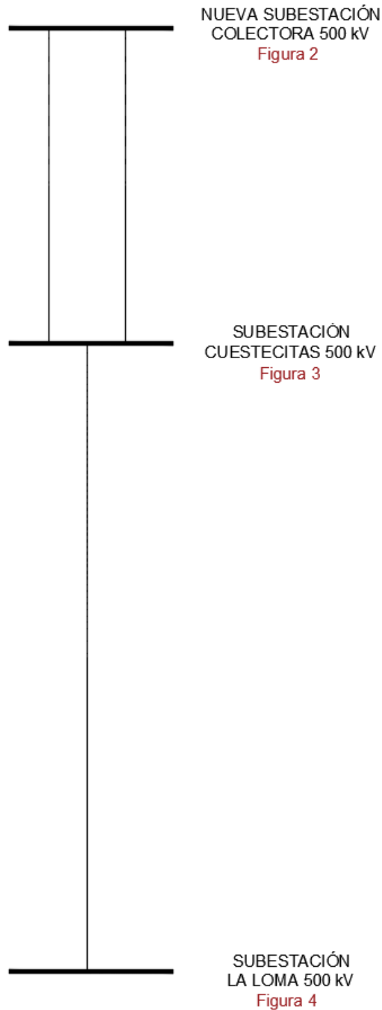
FIGURA 1. DIAGRAMA ESQUEMATICO
