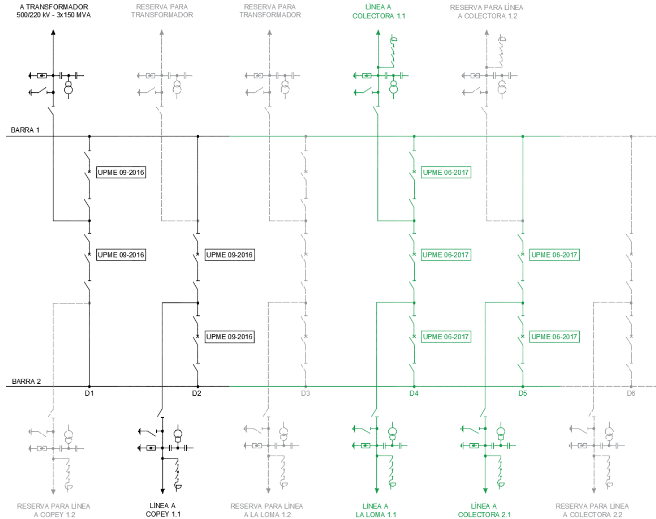
FIGURA 3 CUESTECITAS 500 kV
