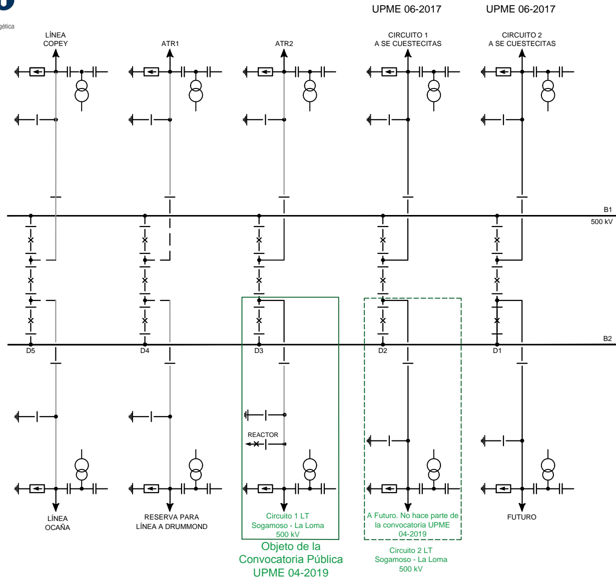
Figura 2. Diagrama Unifilar La Loma 500 kV
