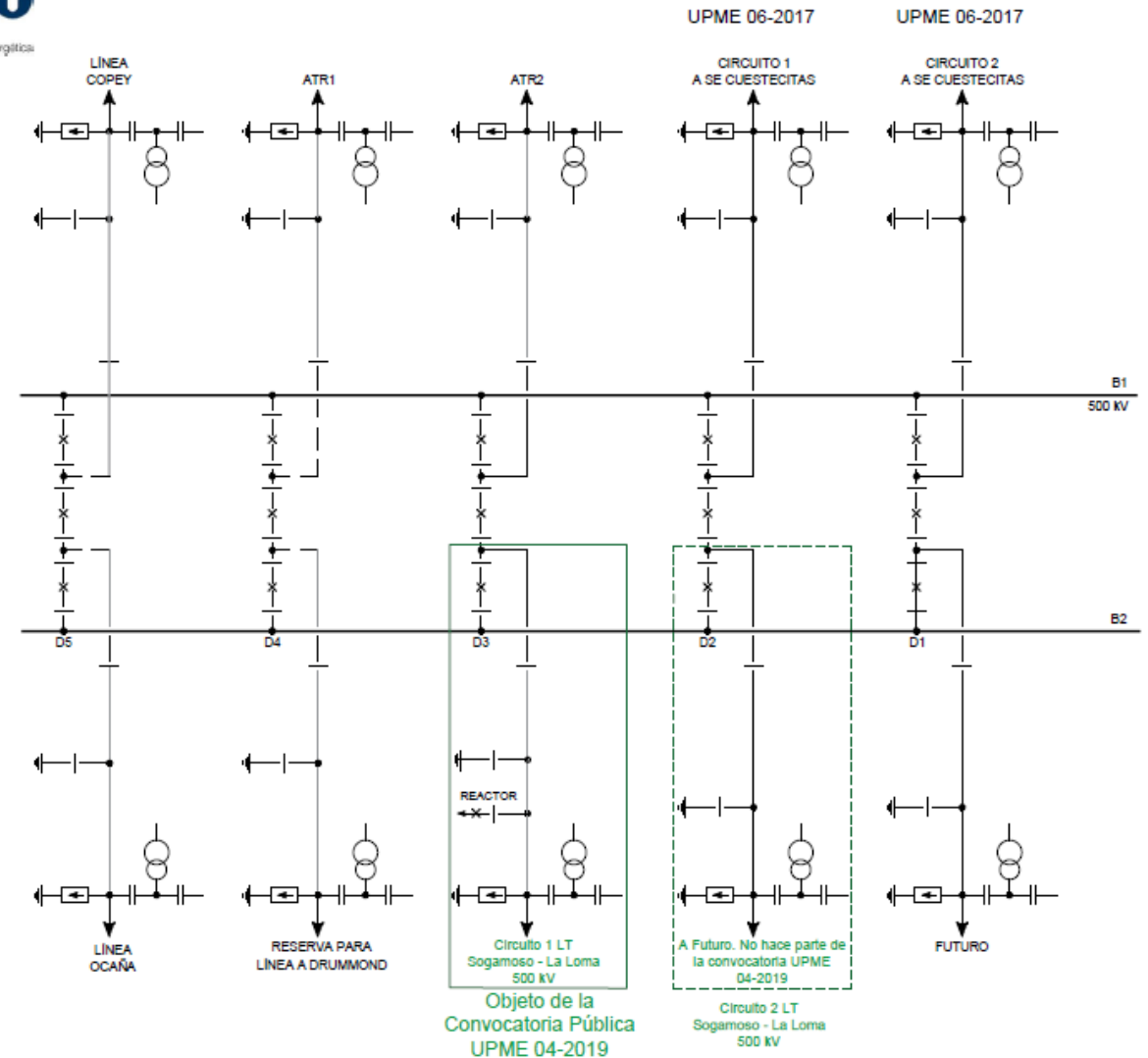
Figura 2. Diagrama Unifilar La Loma 500 kV
