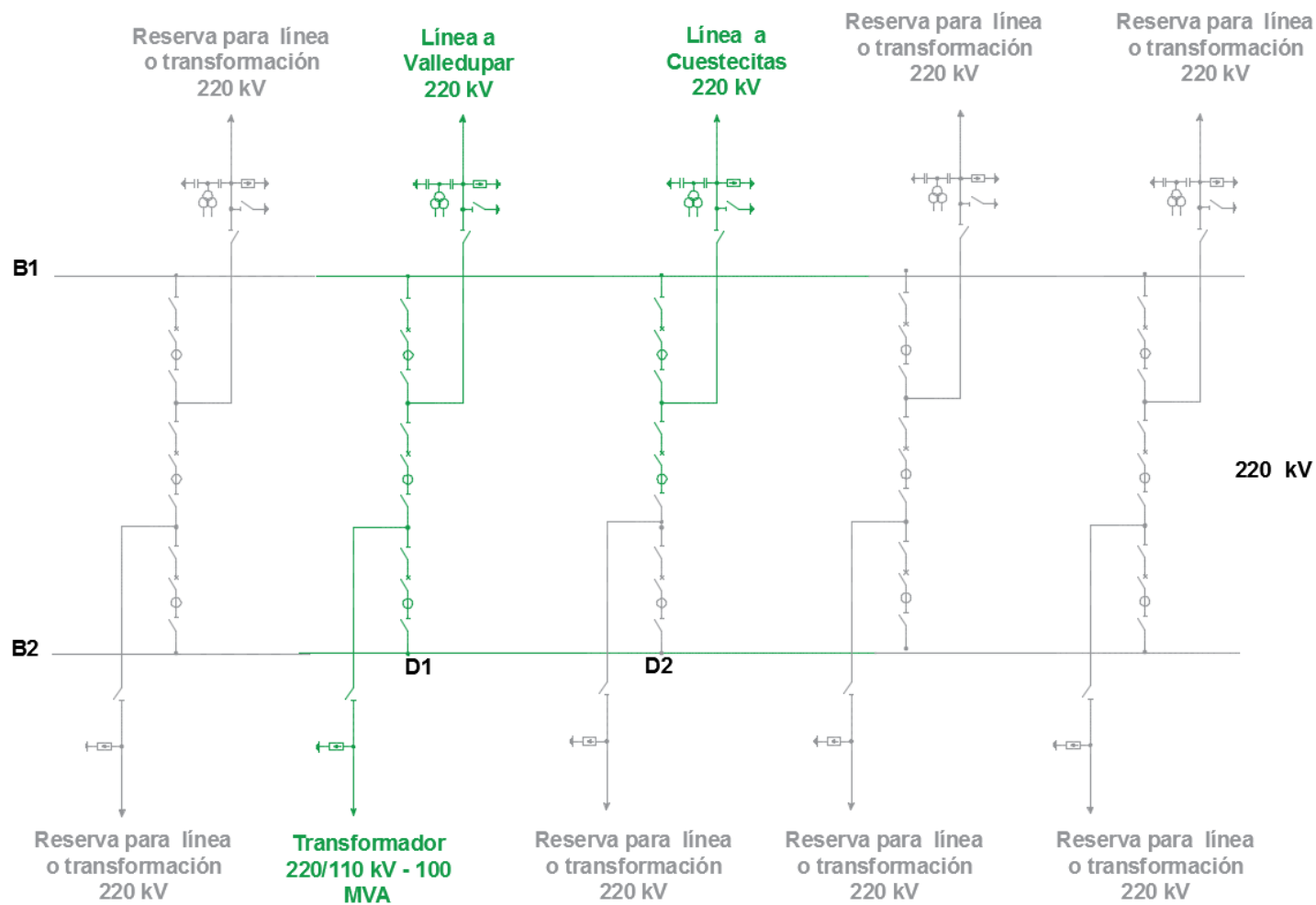
Figura 2 – Diagrama Unifilar Subestación San Juan 220 kV (PREPUBLICACIÓN)
