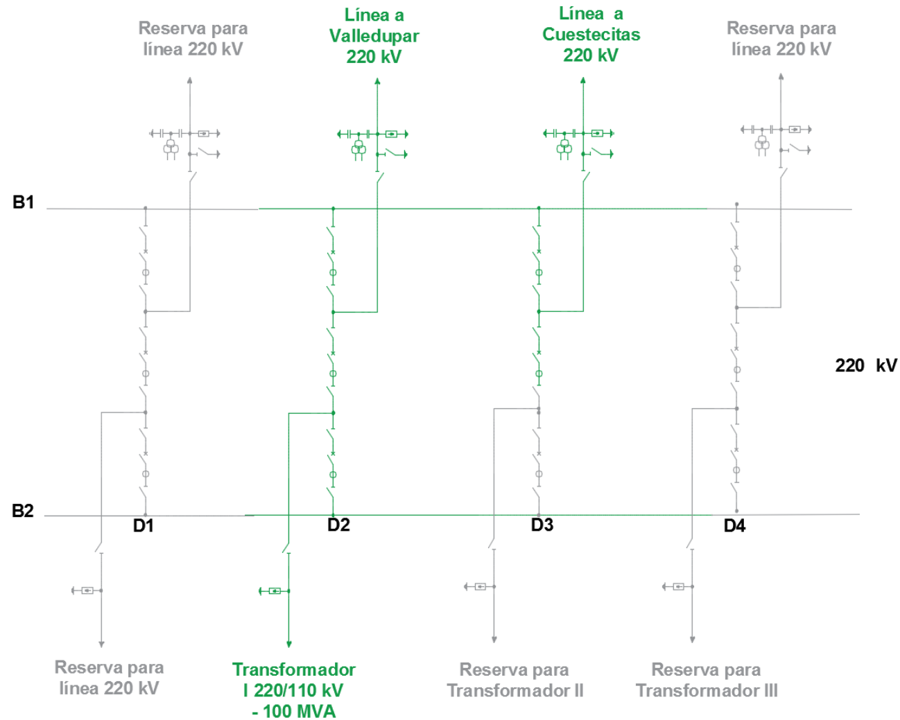
Figura 2 – SE San Juan 220 kV
