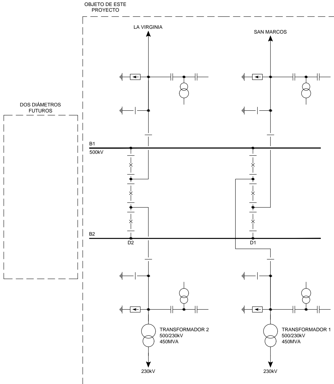
FIGURA 5 ESQUEMA UNIFILAR SUBESTACIÓN ALFEREZ 500kV
