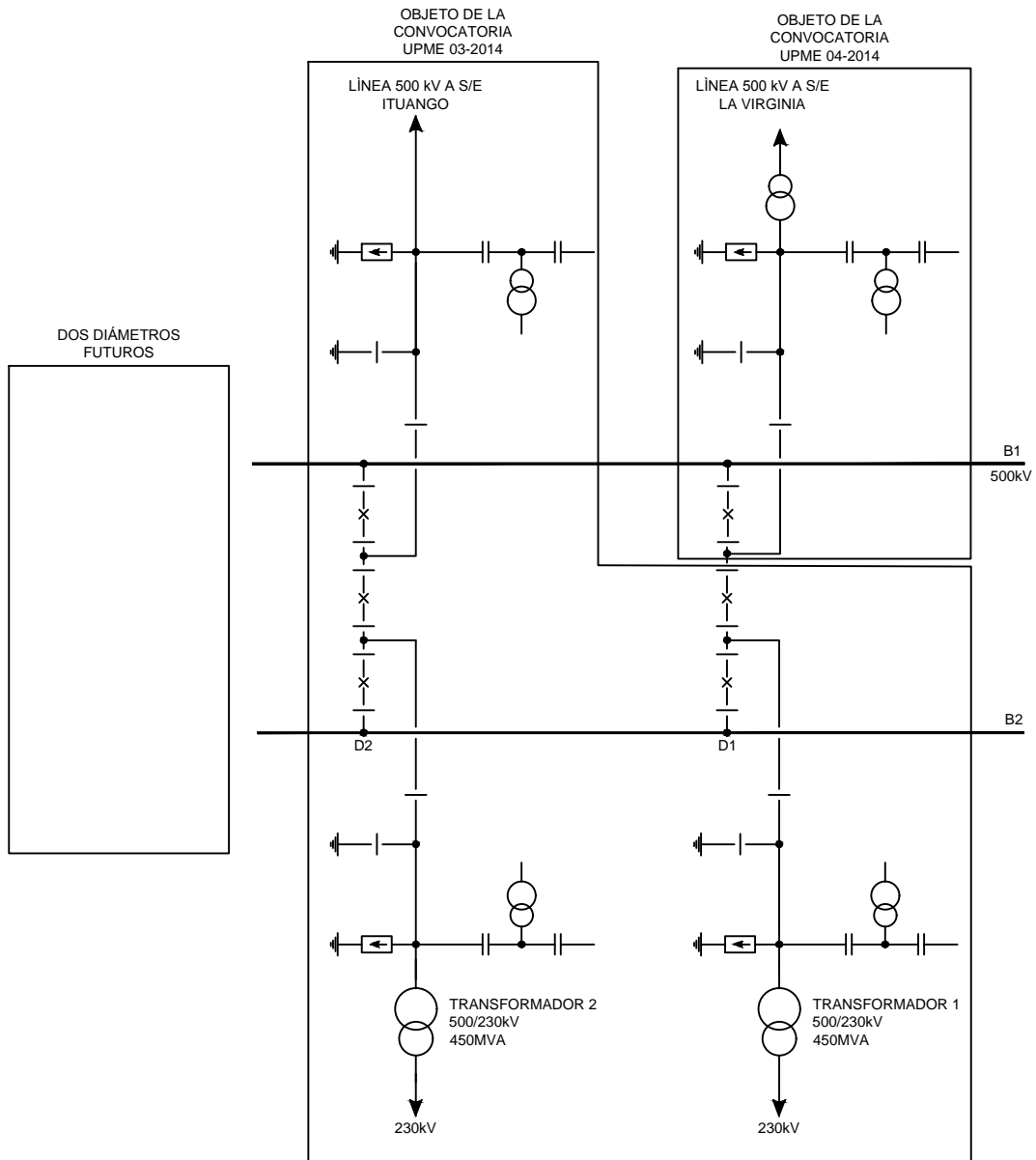
FIGURA 3 ESQUEMA UNIFILAR SUBESTACIÓN MEDELLIN 500 kV
