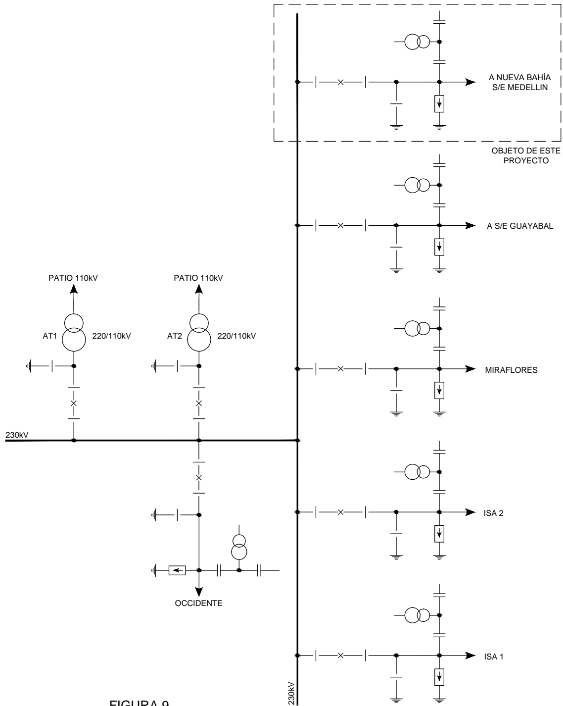
FIGURA 9 ESQUEMA UNIFILAR AMPLIACIÓN DE LA SUBESTACIÓN ANCON SUR 230kV
