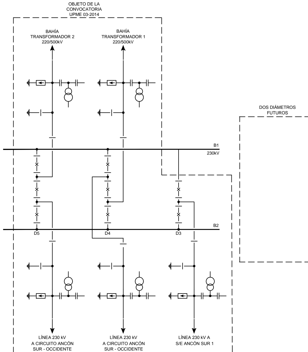
FIGURA 8 ESQUEMA UNIFILAR SUBESTACIÓN MEDELLÍN 230kV
