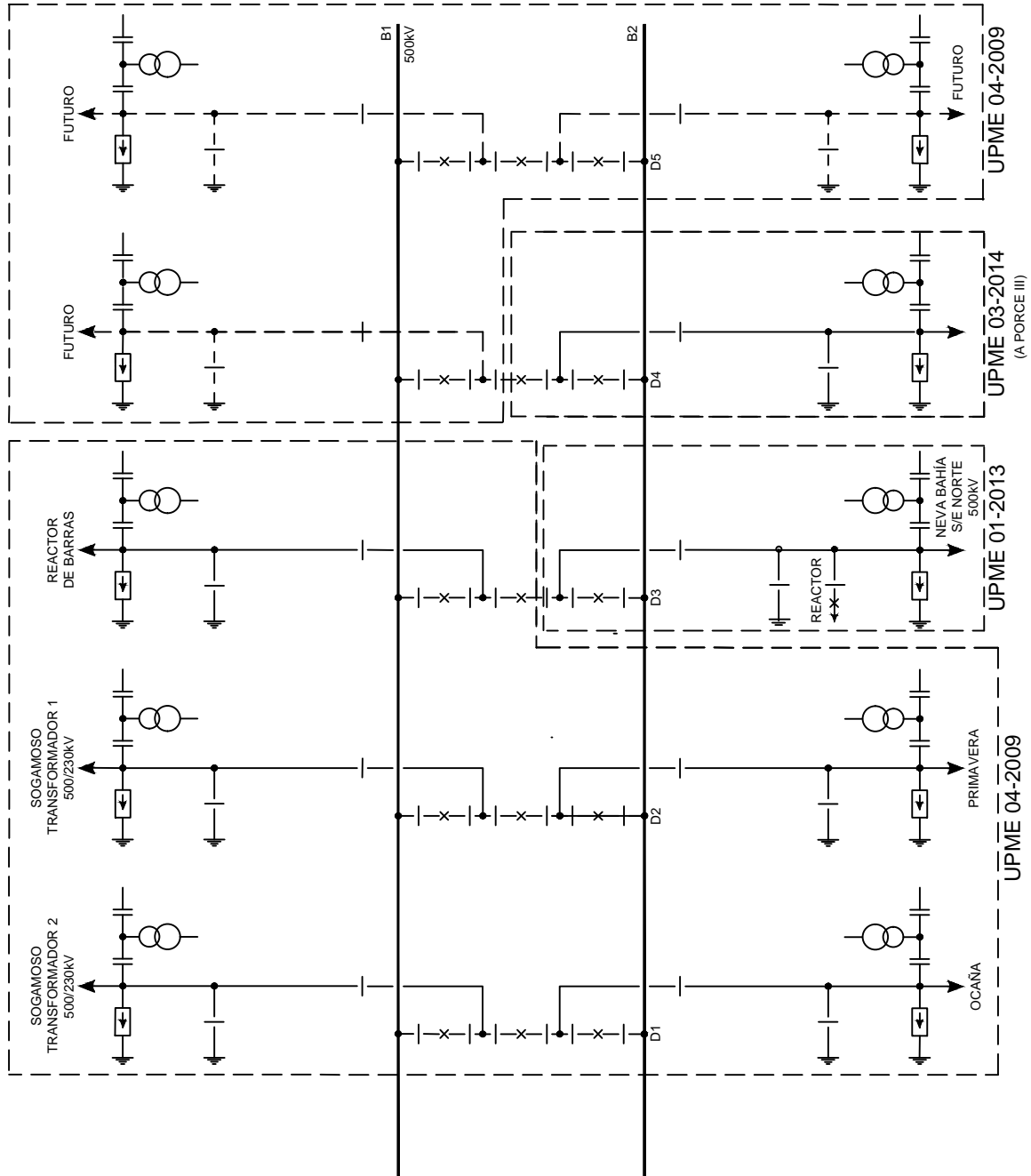
FIGURA 6 ESQUEMA UNIFILAR SUBESTACIÓN SOGAMOSO 500kV
