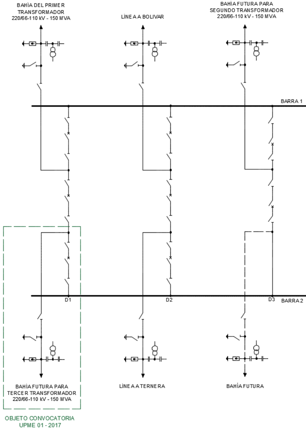
Figura 1. Subestación GIS El Bosque 220 kV
