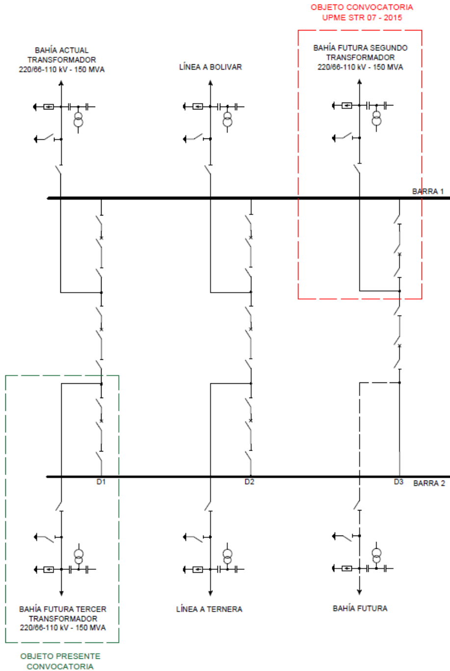
FIGURA 1. ESQUEMA UNIFILAR EXPANSIÓN SUBESTACIÓN GIS EL BOSQUE 220 kV
