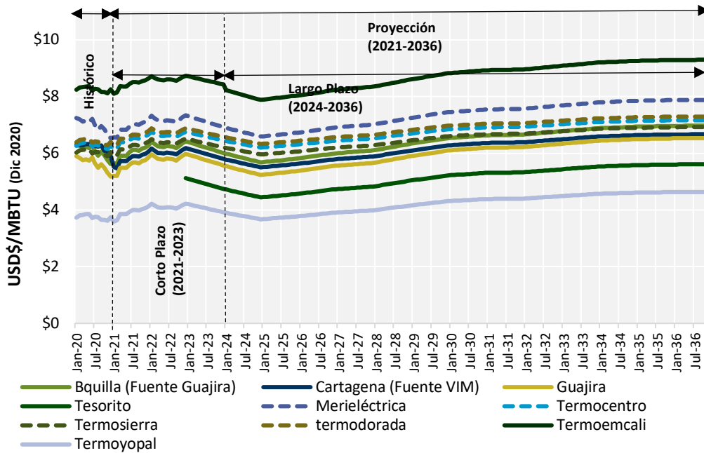
Gráfica 13 Proyección de precios de gas en plantas termoeléctricas
