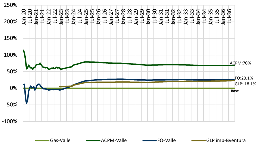
Gráfica 4. Precios relativos para generación en el suroccidente
