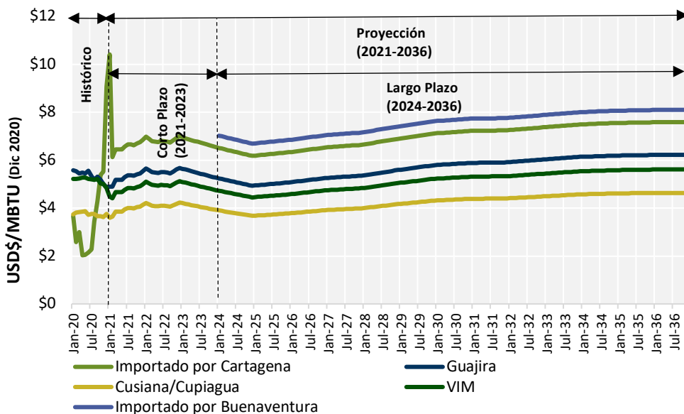
Gráfica 5 Proyección de precios de gas natural en fuente de producción
