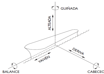
Figura 2. Movimientos del buque en sus 6 grados de libertad
