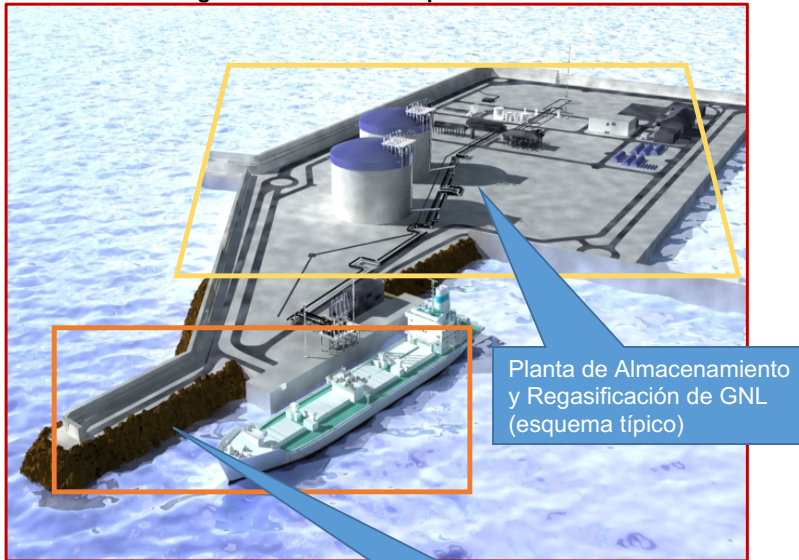
Figura 3. Subsistemas opción en tierra
