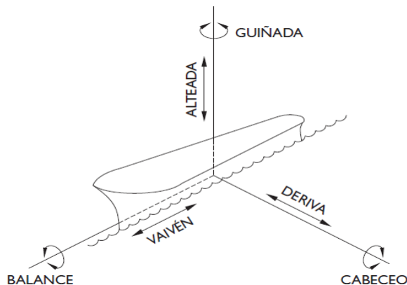
29 30 Figura 2. Movimientos del buque en sus 6 grados de libertad
