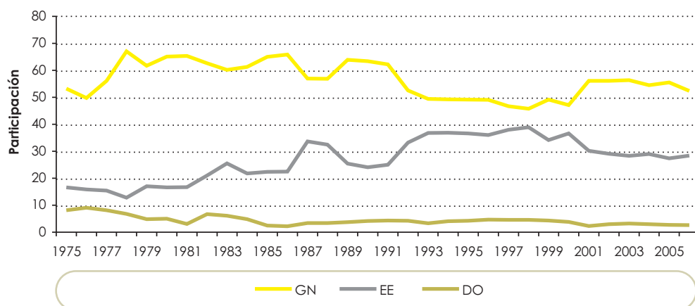
Gráfica 63 CONSUMO DE ENERGÍA EN EL SECTOR INDUSTRIAL Maderas y Muebles
