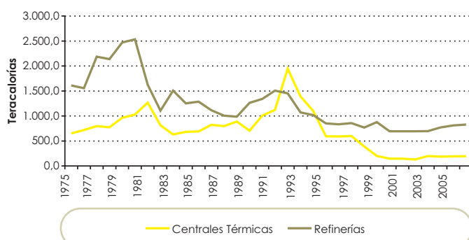
Grafico 32 CONSUMO PROPIO CENTROS DE TRANSFORMACIÓN
