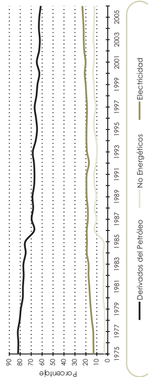
Gráfica 21 CONSUMO FINAL DE ENERGÍA SECUNDARIA Participaciones
