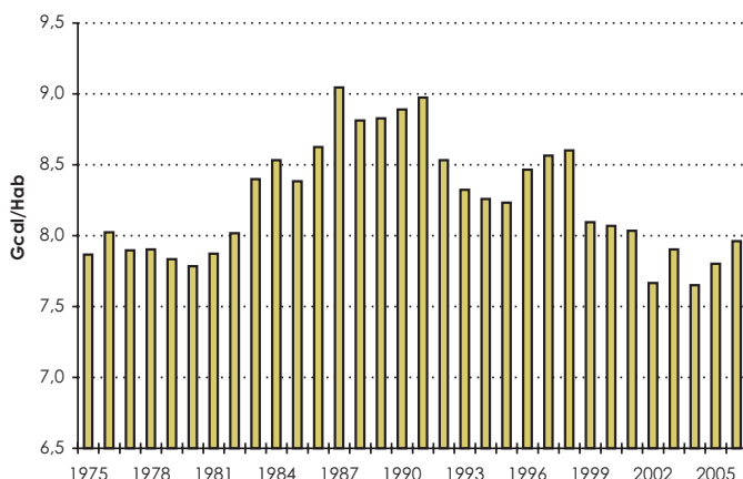
Gráfica 41 OFERTA INTERNA DE ENERGÍA PER CÁPITA
