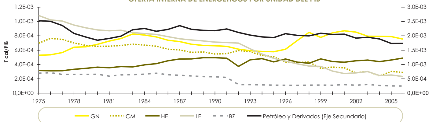
Gráfica 43 OFERTA INTERNA DE ENERGÉTICOS POR UNIDAD DEL PIB
