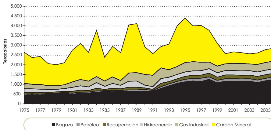
Gráfica 34 AUTOGENERACIÓN DE ELECTRICIDAD POR ENERGÉTICO
