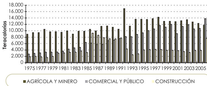
Gráfica 30 CONSUMO FINAL SECTORIAL
