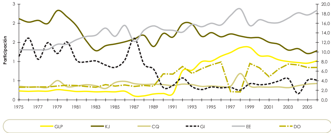
Gráfica 58 CONSUMO DE ENERGÍA EN EL SECTOR INDUSTRIAL
