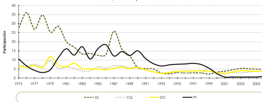
Gráfica 68 CONSUMO DE ENERGÍA EN EL SECTOR INDUSTRIAL Hierro, Acero y No Ferrosos
