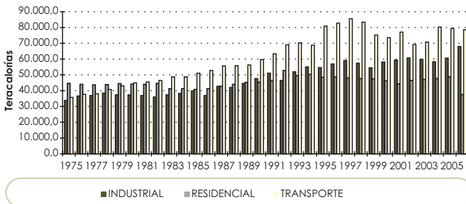
Gráfica 28 CONSUMO FINAL SECTORIAL
