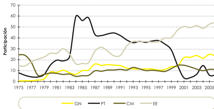
Gráfica 62 CONSUMO FINAL EN EL SECTOR INDUSTRIAL Calzado y Cueros
