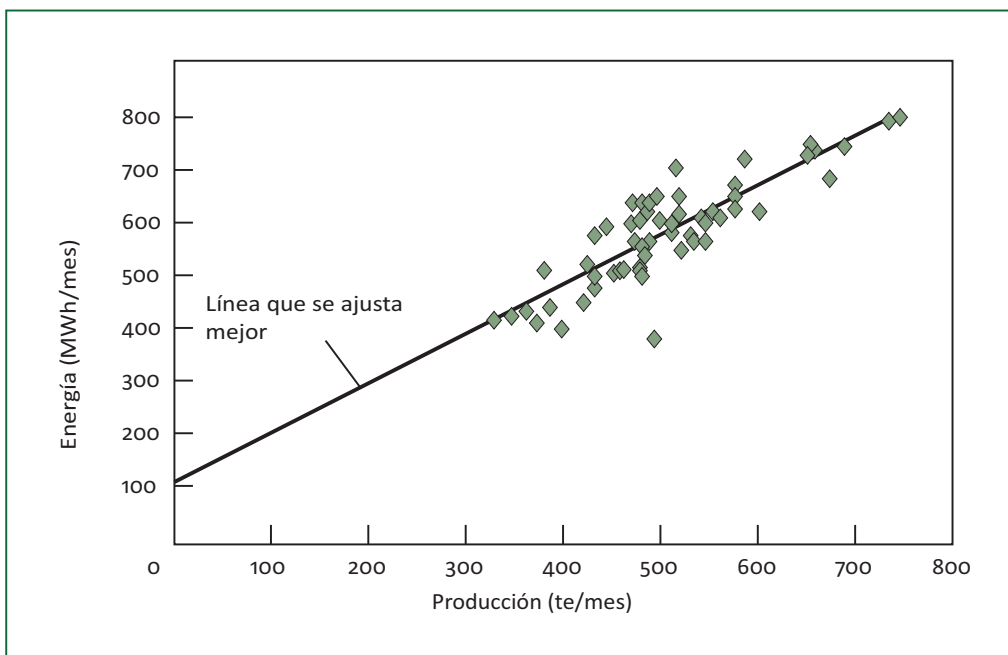
Figura XVI Gráfico que representa los datos medidos incluida la línea que se ajusta mejor
