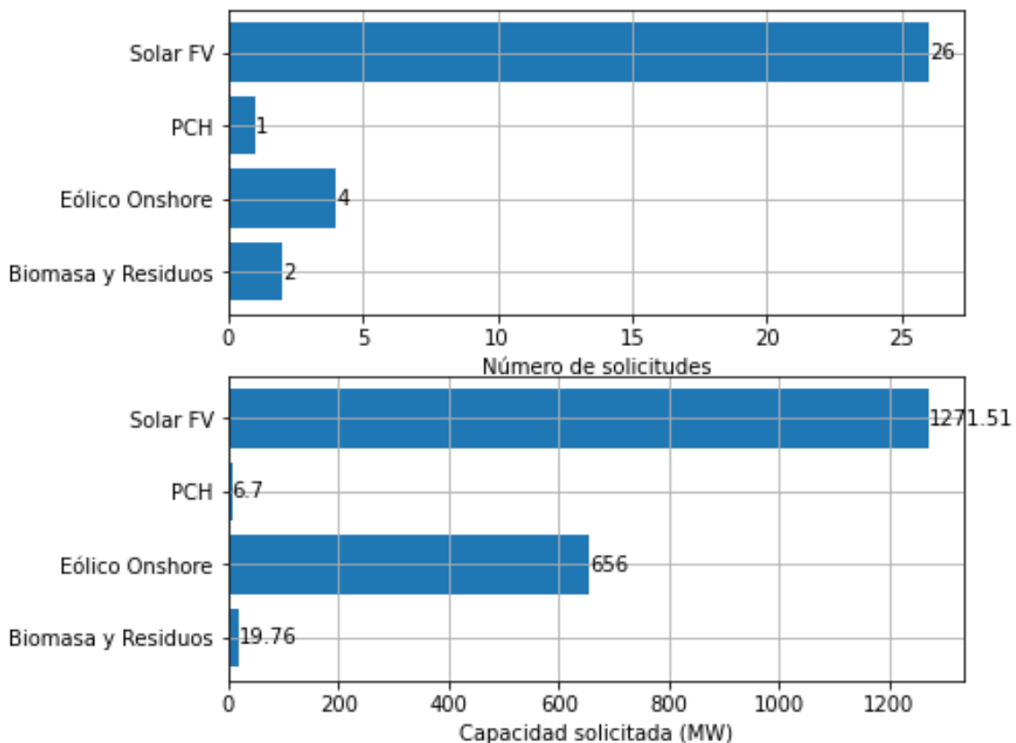
Figura 1. Número de solicitudes y capacidad solicitada por tecnología en la subárea Oriental.
