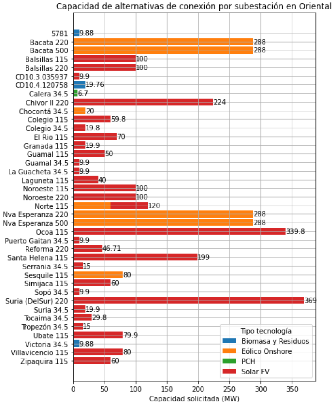
Figura 3. Número de solicitudes por subestación en la subárea Oriental.
