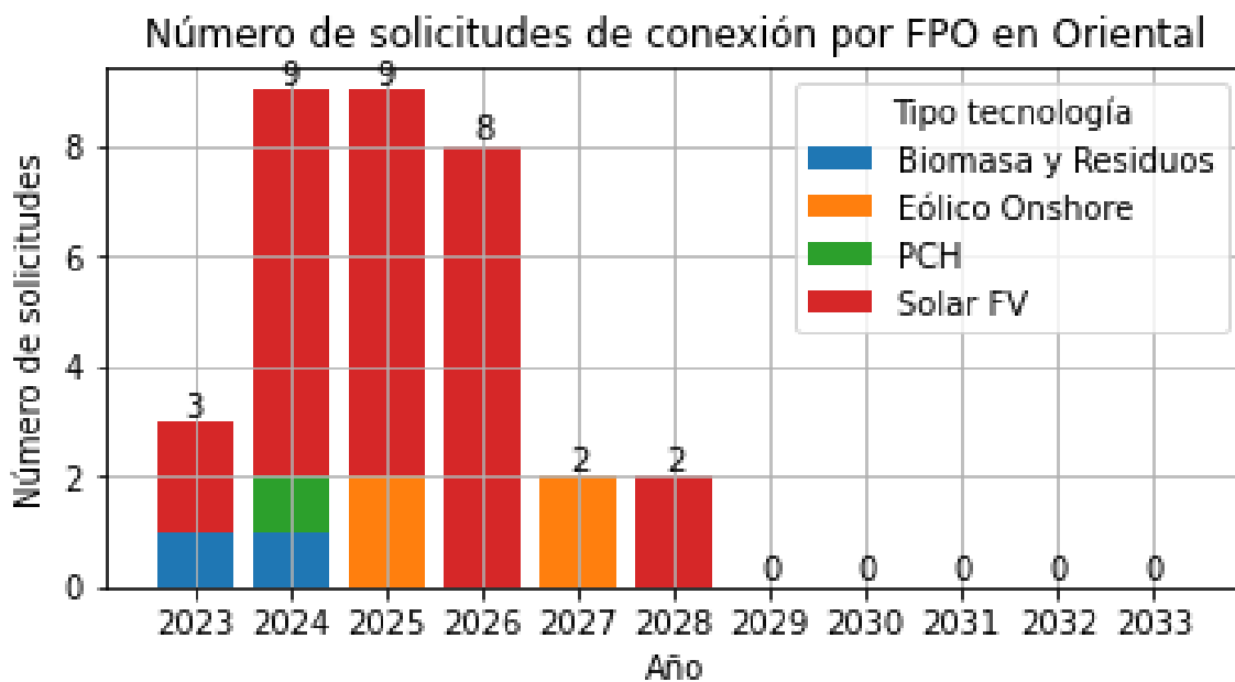
Figura 4. Número de solicitudes de conexión por FPO en Oriental
