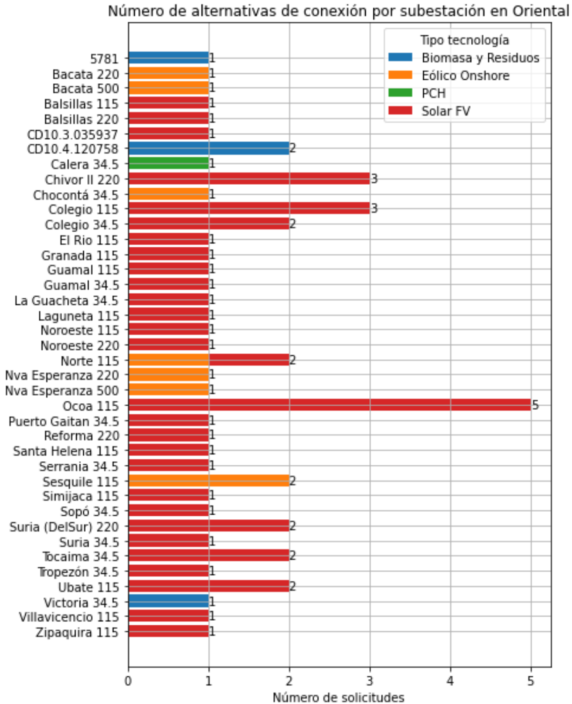
Figura 2. Número de solicitudes por subestación en la subárea Oriental.
