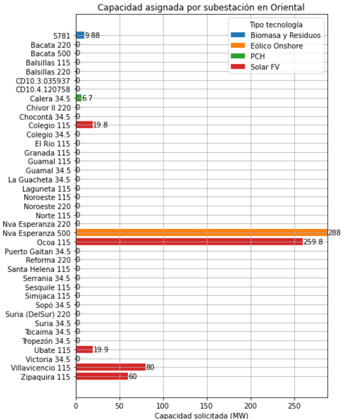
Figura 8. Capacidad de proyectos asignados por subestación en Oriental.
