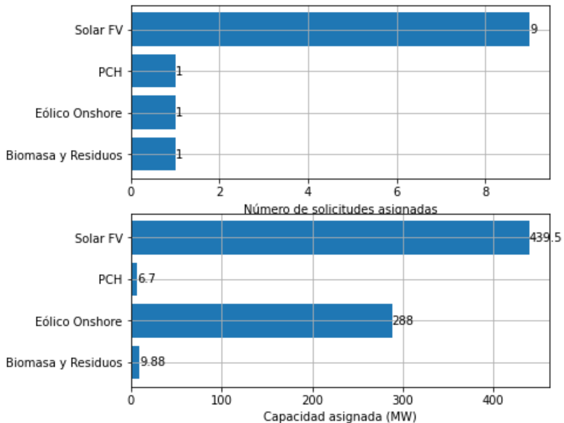
Figura 6. Número de solicitudes y capacidad asignada por tecnología en la subárea Oriental.
