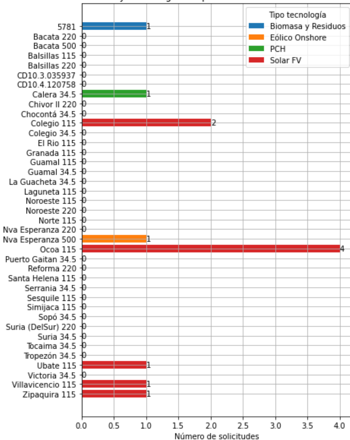
Figura 7. Número de proyectos asignados por subestación en Oriental.
