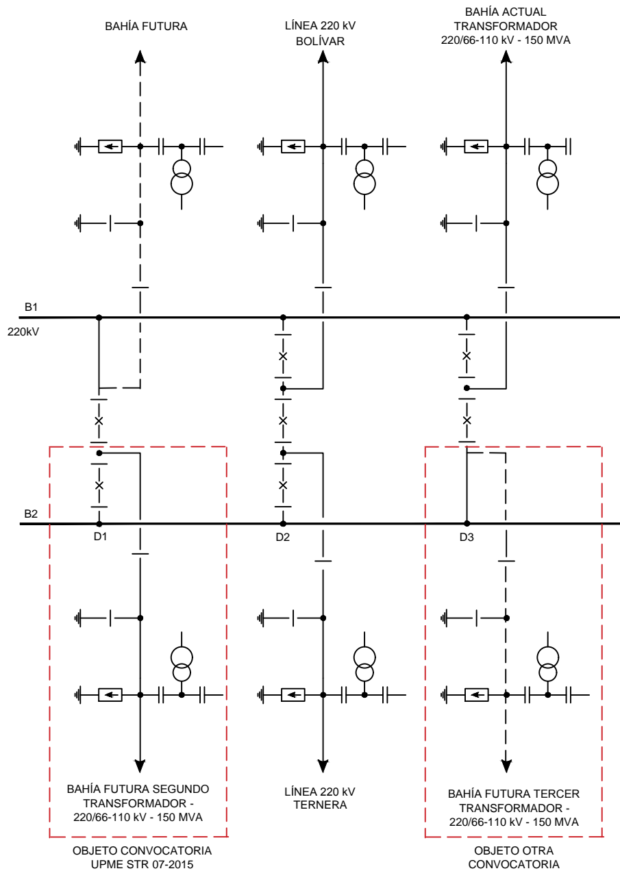
FIGURA 1. ESQUEMA UNIFILAR EXPANSIÓN SUBESTACIÓN BOSQUE 220 kV
