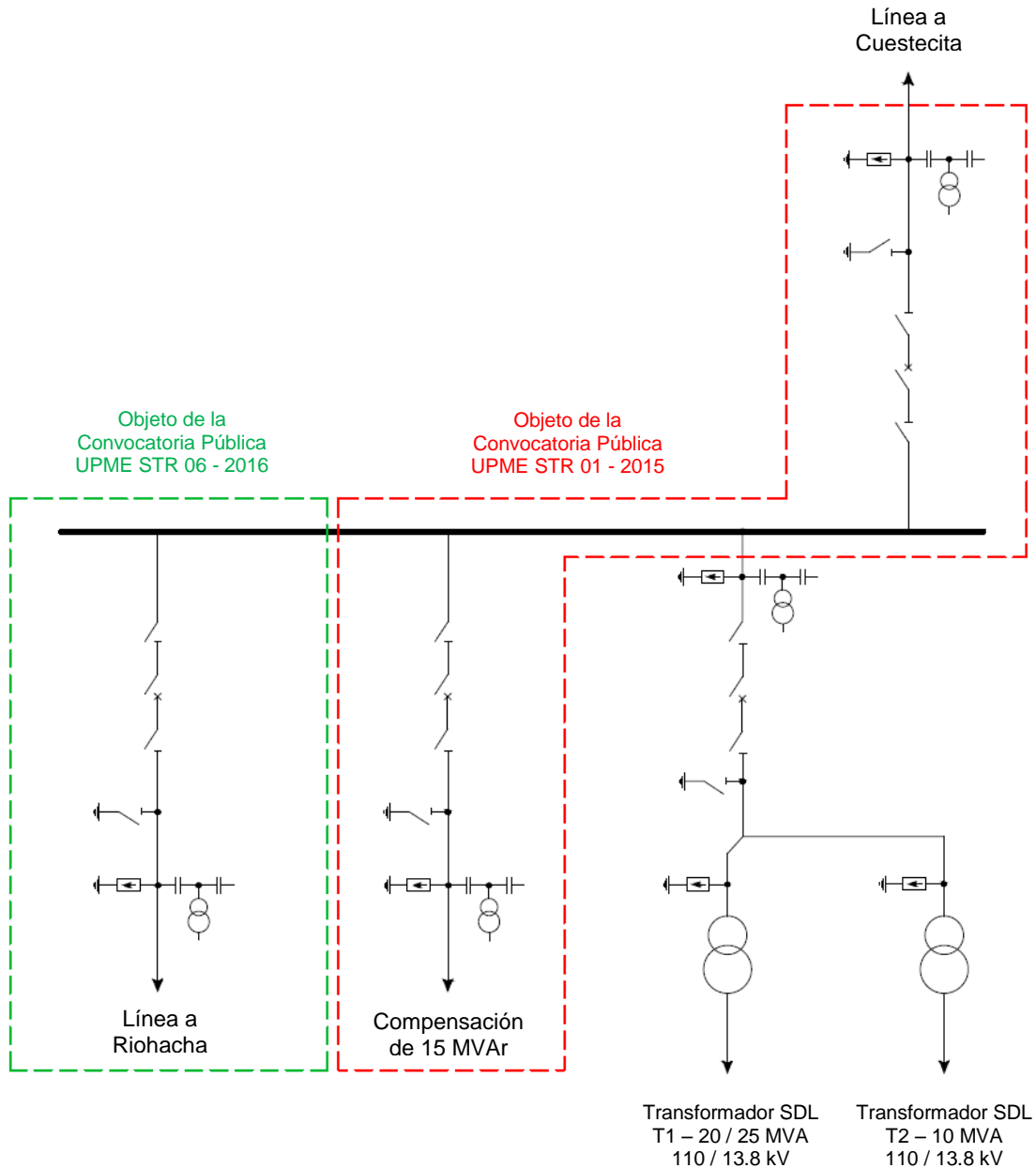
FIGURA 3. ESQUEMA UNIFILAR SUBESTACIÓN MAICAO 110 kV
