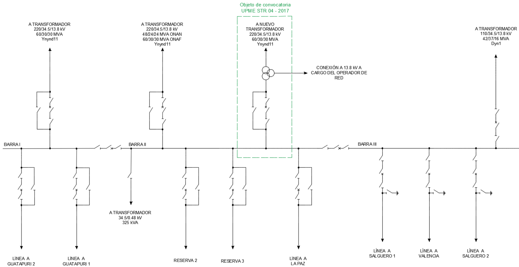
FIGURA 1. SUBESTACIÓN VALLEDUPAR 34.5 kV
