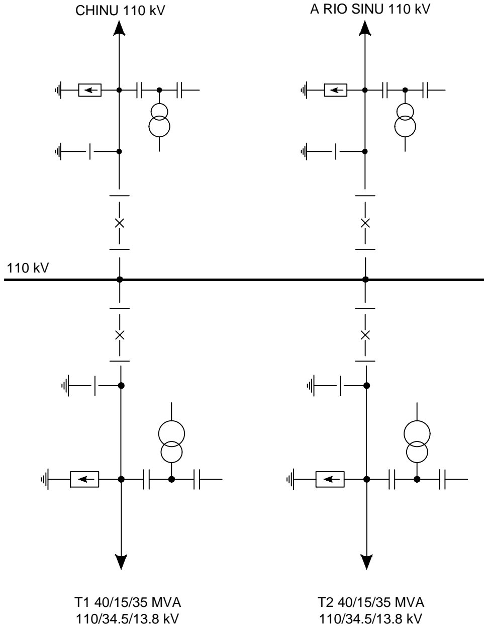
FIGURA 3 ESQUEMA UNIFILAR SUBESTACIÓN MONTERÍA 110 kV
