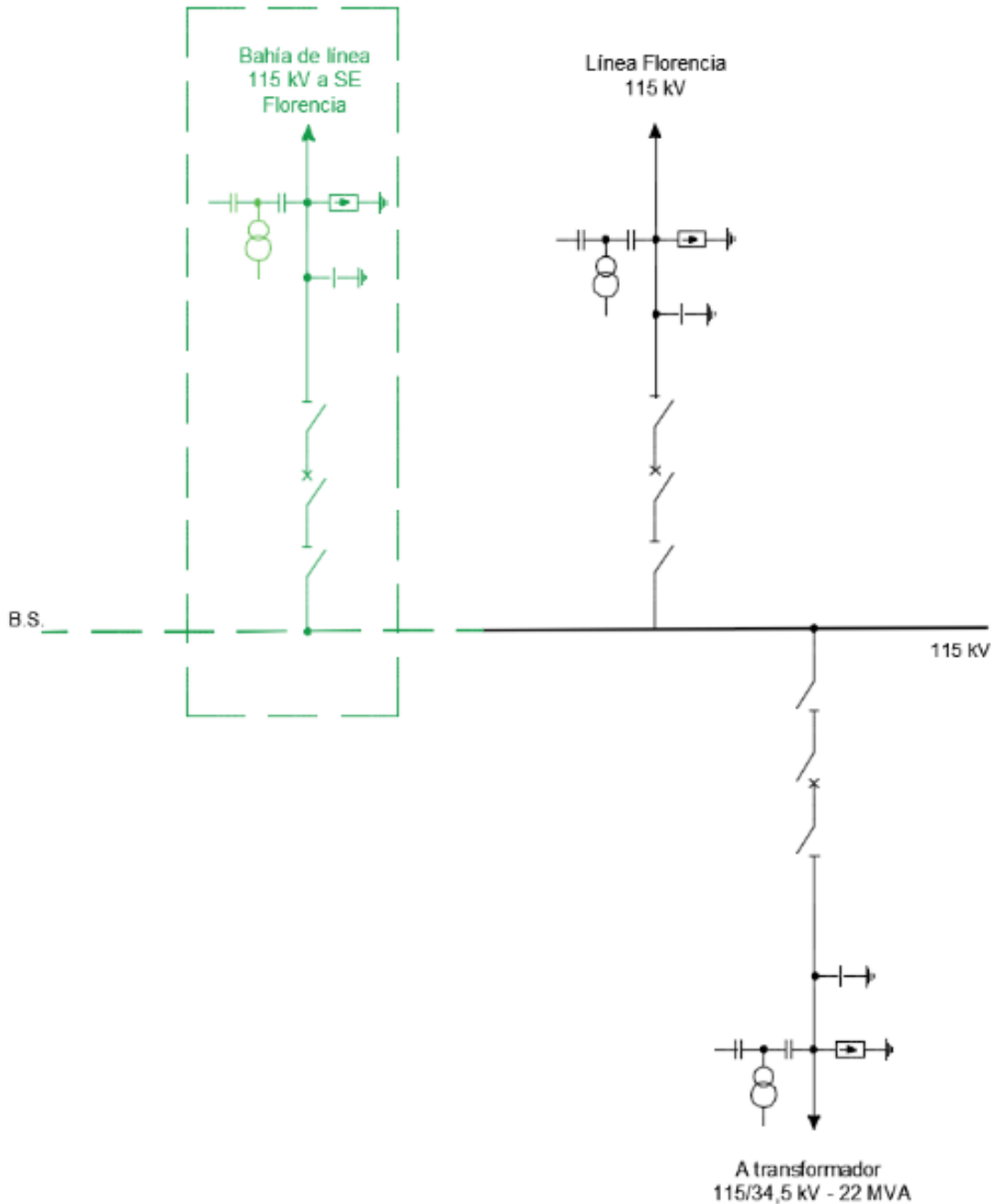
FIGURA 4. ESQUEMA UNIFILAR SUBESTACIÓN DONCELLO 115 kV (PREPUBLICACIÓN)
