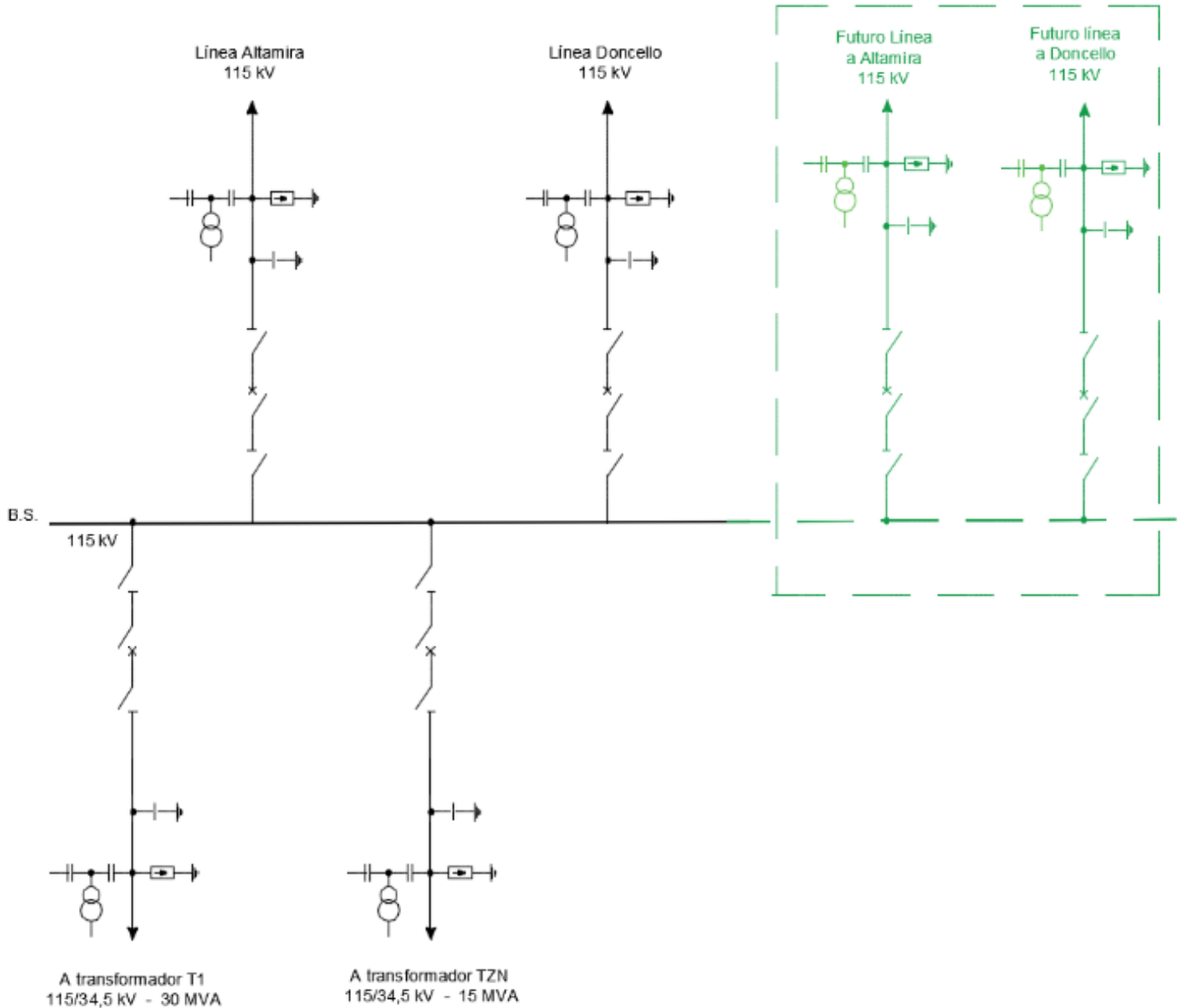
FIGURA 3. ESQUEMA UNIFILAR SUBESTACIÓN FLORENCIA (centro) 115 kV (PREPUBLICACIÓN)
