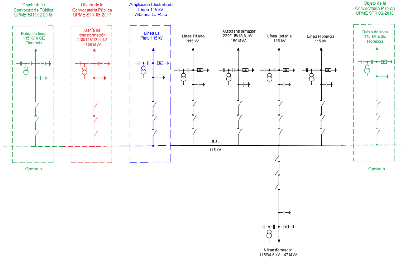
FIGURA 2. ESQUEMA UNIFILAR SUBESTACIÓN ALTAMIRA 115 kV (PREPUBLICACIÓN)
