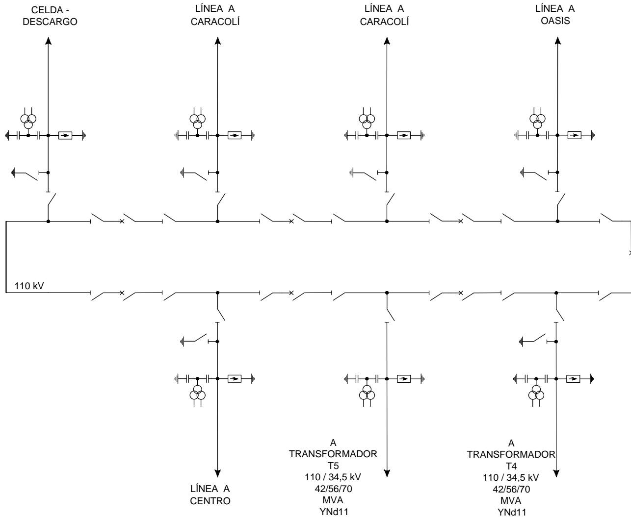
Figura 3. Diagrama Unifilar subestación Silecio 110 kV (Prepublicación)
