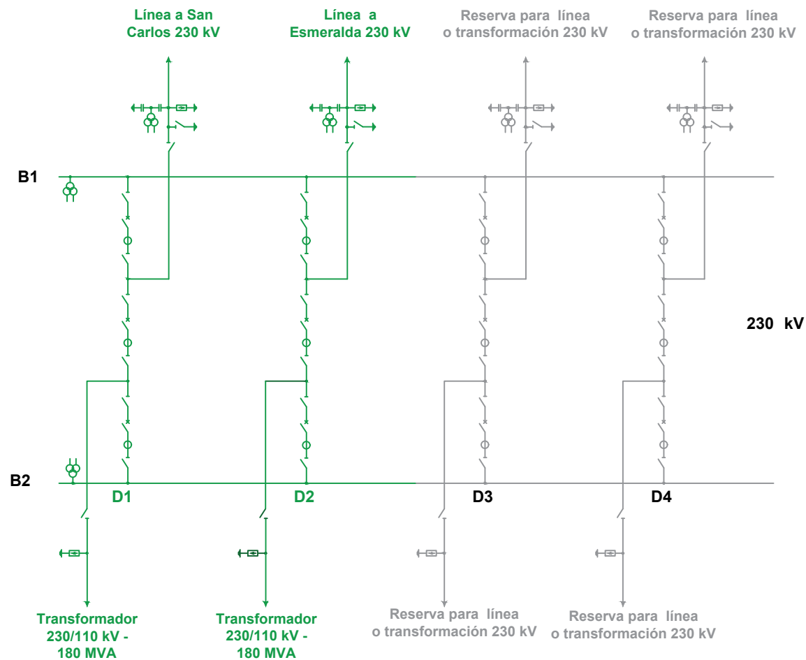
Figura 2. Diagrama Unifilar Corrientes 230 kV
