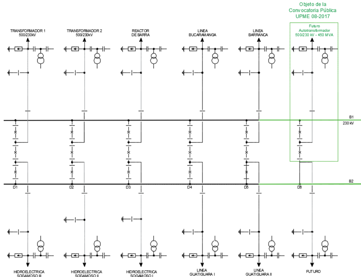
Figura 2 - Diagrama Unifilar Subestación Sogamoso 230 kV
